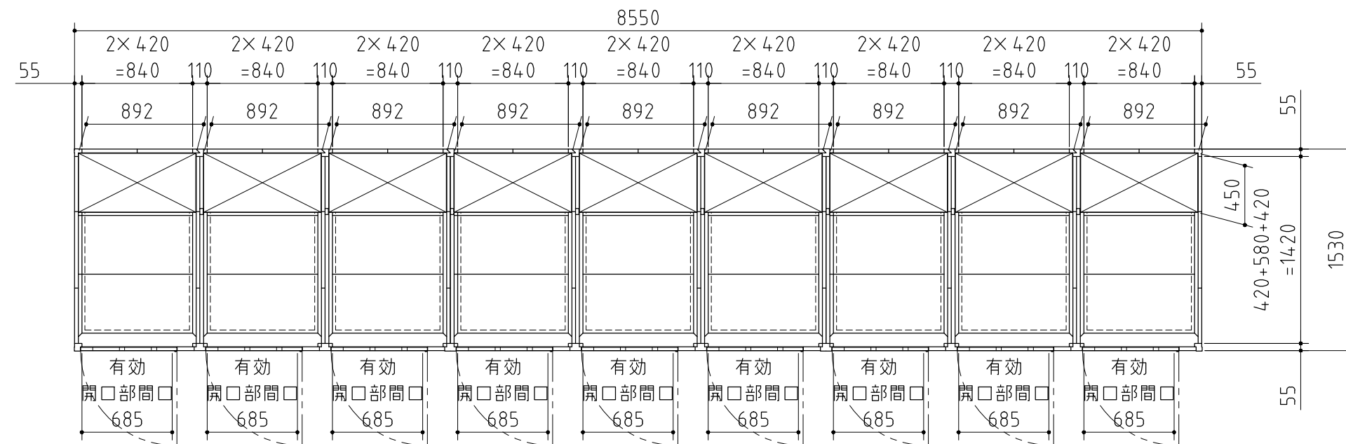
平面図
